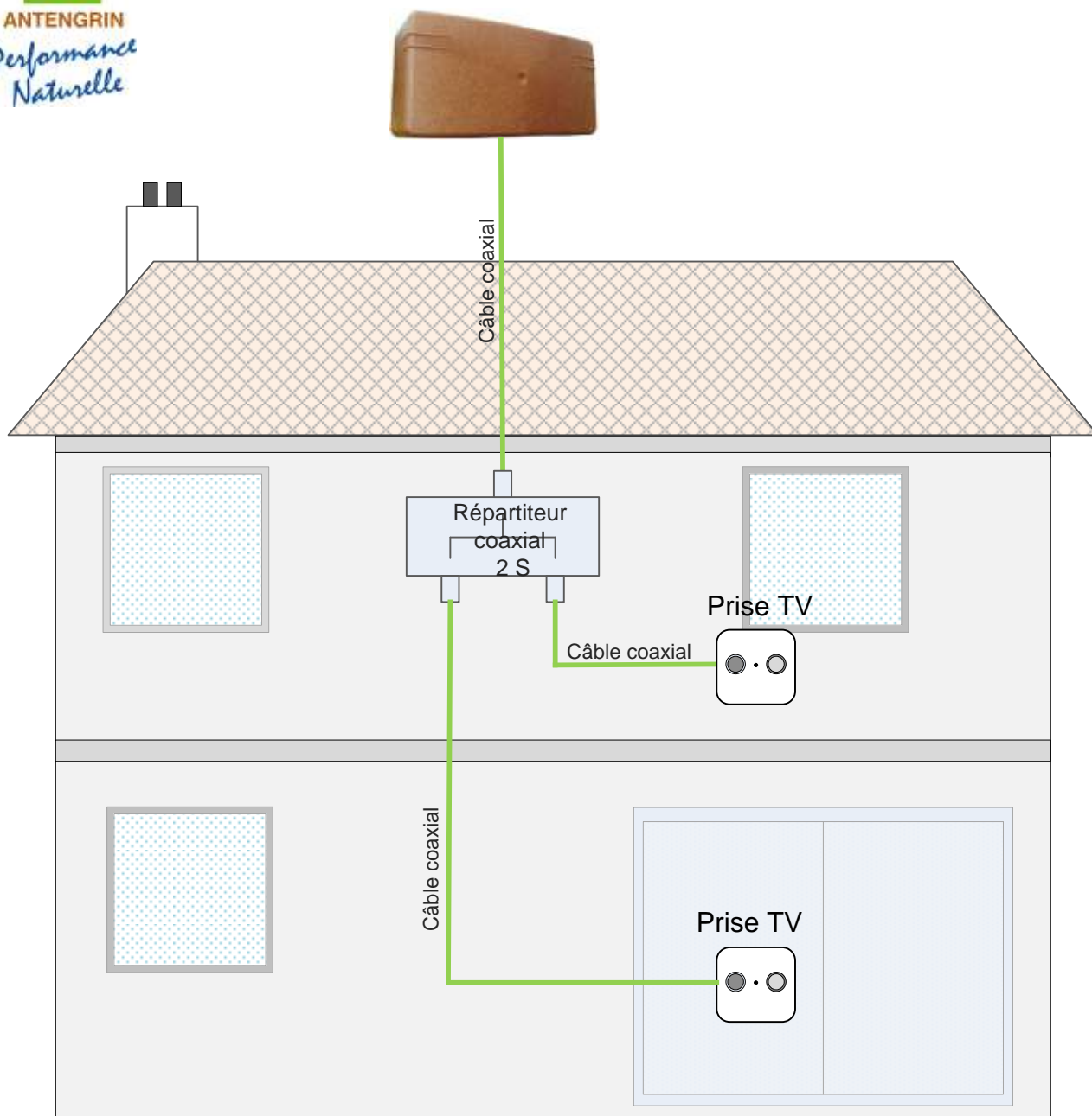
Configuration simplifiée sur deux prises ( sans Amplificateur )
