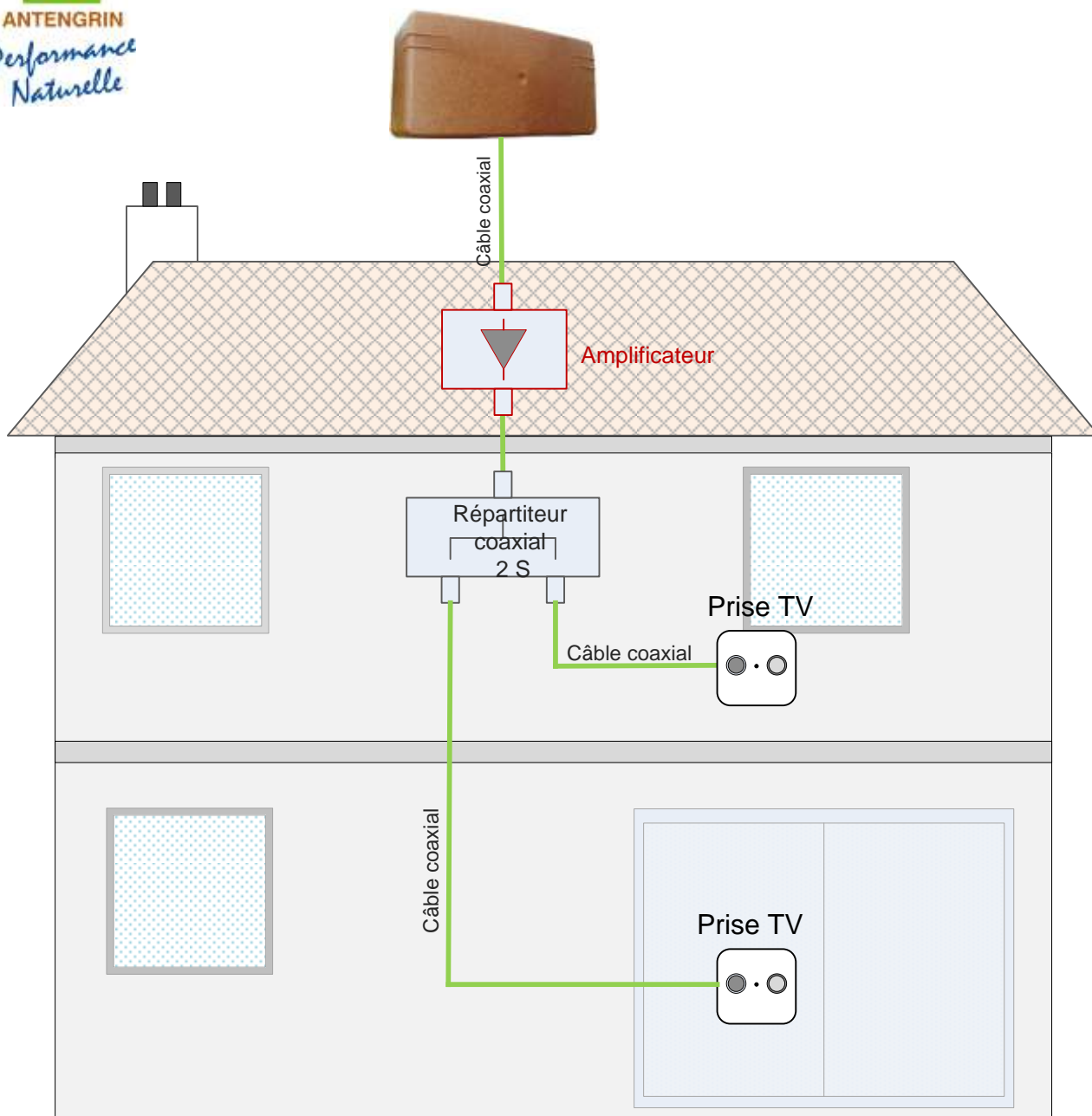
Configuration sur deux prises avec Amplificateur de faible bruit Conseillée dans des conditions de réception défavorable
